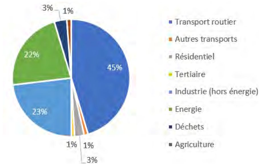
Figure 4 : Répartition des émissions de NOx dans la CC d'Entre Bièvre et Rhône en 2019 (Source : Atmo Auvergne-Rhône-Alpes, Diagnostic territorial)
